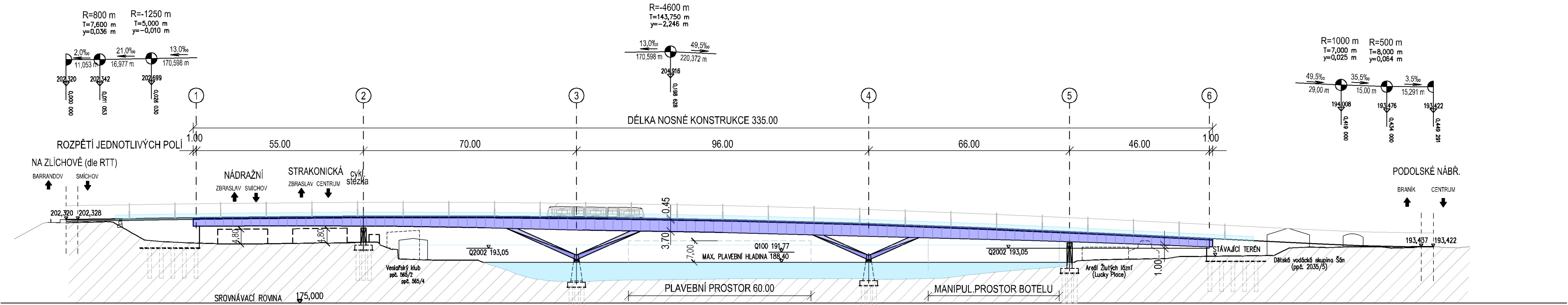
Podélný řez 1:1000
