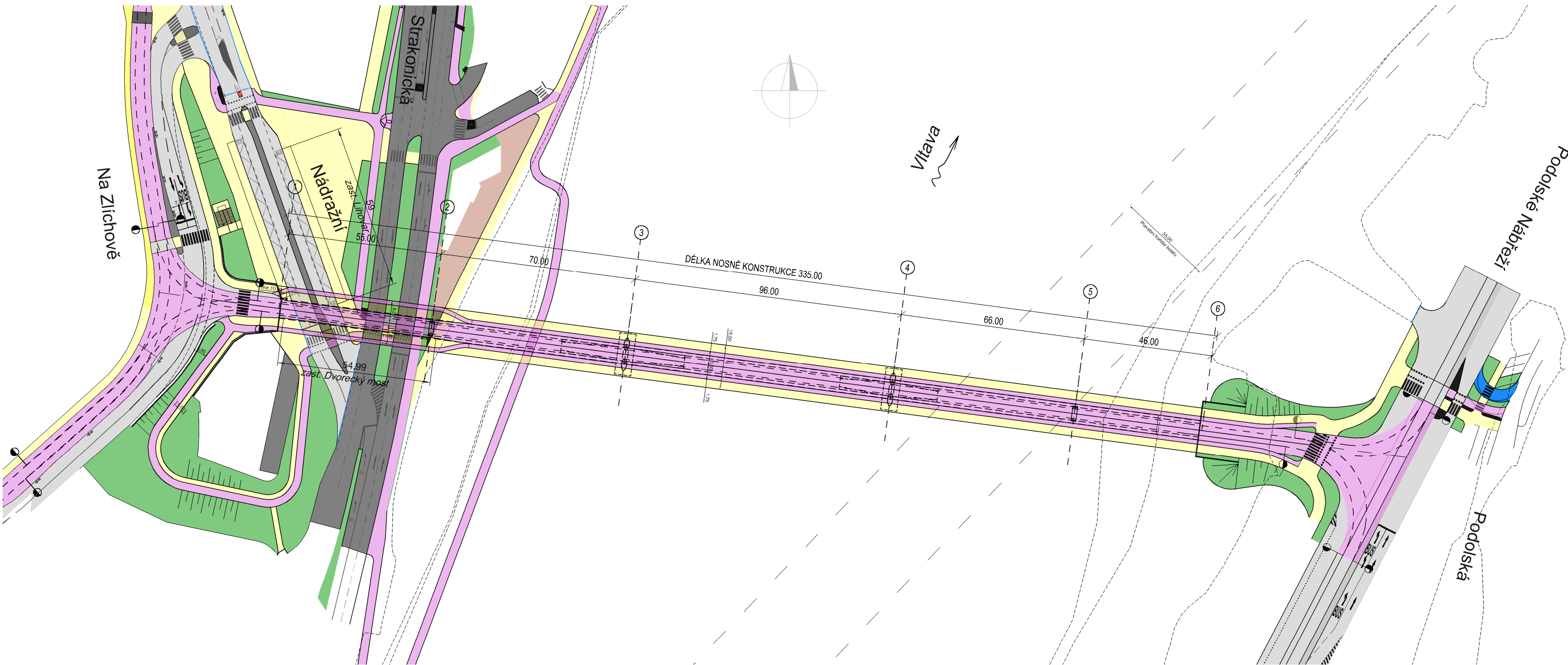
Situace 1:1000
